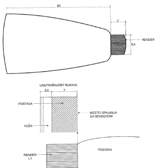
Слика 3: Приказ унутрашњости (постава) рукава
