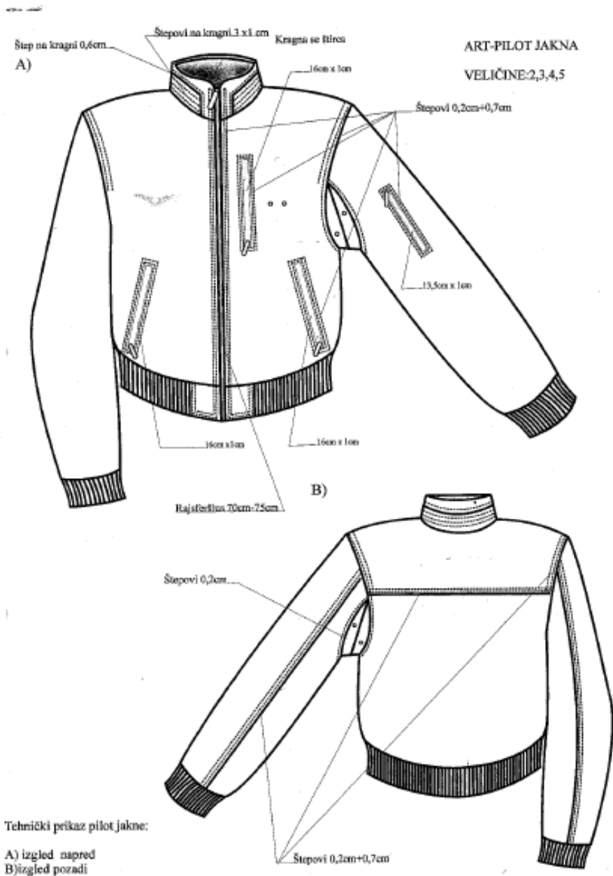
Слика 1: Изглед пилотске кожне јакне
